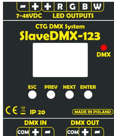
Rysunek 1: Widok panelu sterownika
