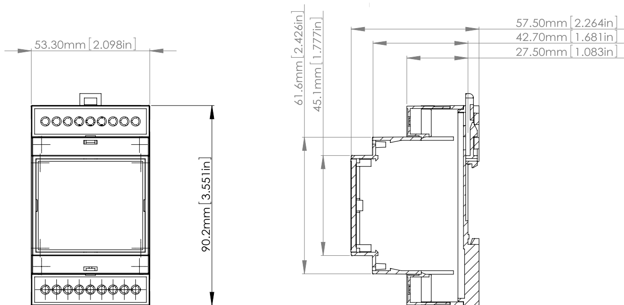
Rysunek 8: Wymiary urządzenia
